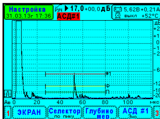
Усиление 17 дБ
