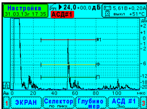
Усиление 24 дБ
