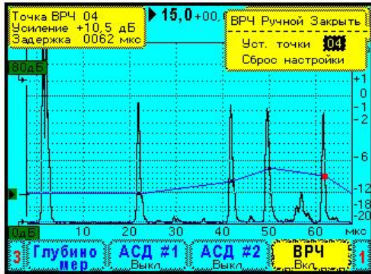
ВРЧ. Стиль "Ручной". Выравнивание амплитуд эхосигналов от отражателей, расположенных на различной глубине в образце
