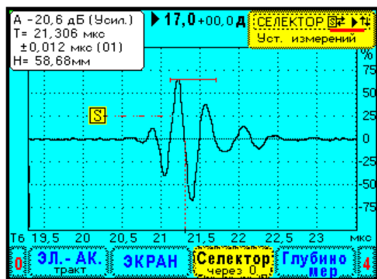
Прецизионные измерения задержки и толщины изделия методом перехода через ноль.
